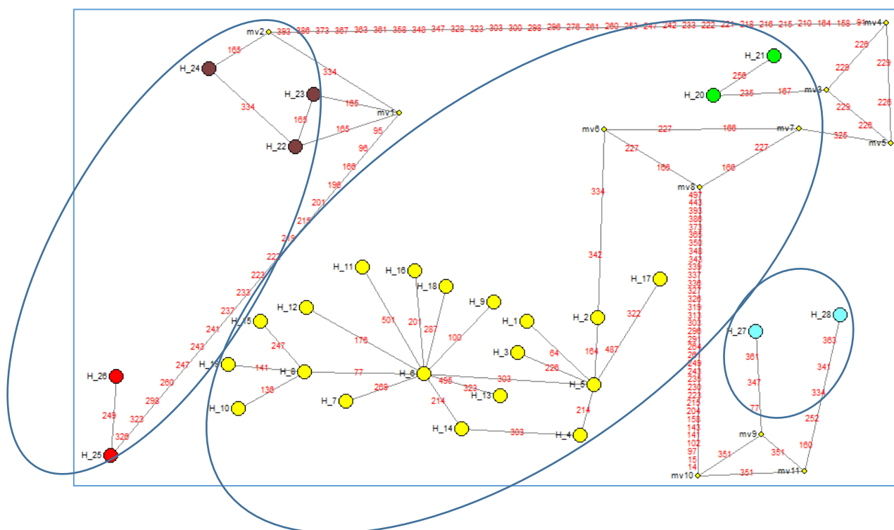
Figura 4. Rede de haplótipos gerada pelo programa network, mostrando as espécies identificadas pelo gene rRN16S. As cores representam as espécies da seguinte forma: vinho= R. mirandaribeiroi ; Amarelo= R. schneideri ; Vermelho; R. granulosa ; Azul claro= R. margaritifera ; Verde= R. marina .
