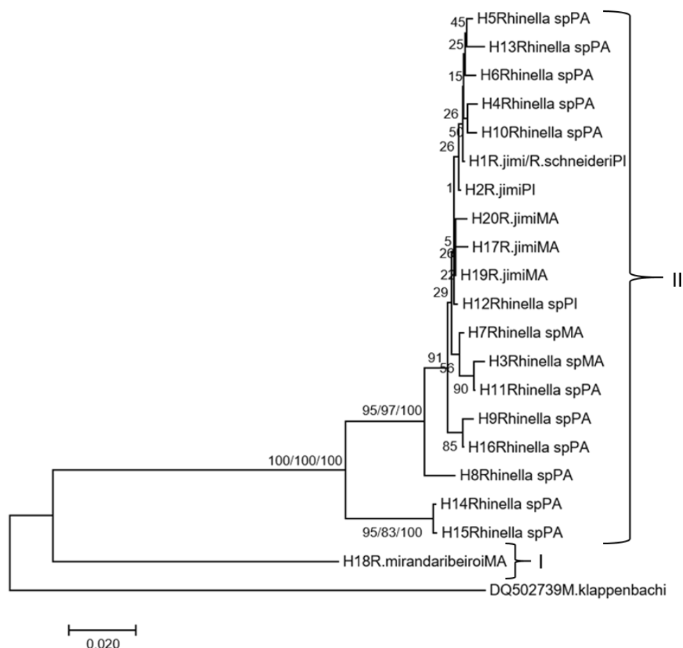
Figura 5. Árvore filogenética obtida através da abordagem de agrupamento de vizinhos (NJ) usando o algoritmo Tamura-3 Parâmetro para haplótipos do gênero Rhinella do meio norte do Brasil, com base no gene COI. Os valores de bootstrap estão na seguinte ordem: Máxima Verossimilhança (ML), Máxima Parcimônia e Agrupamento de Vizinhos (NJ).
