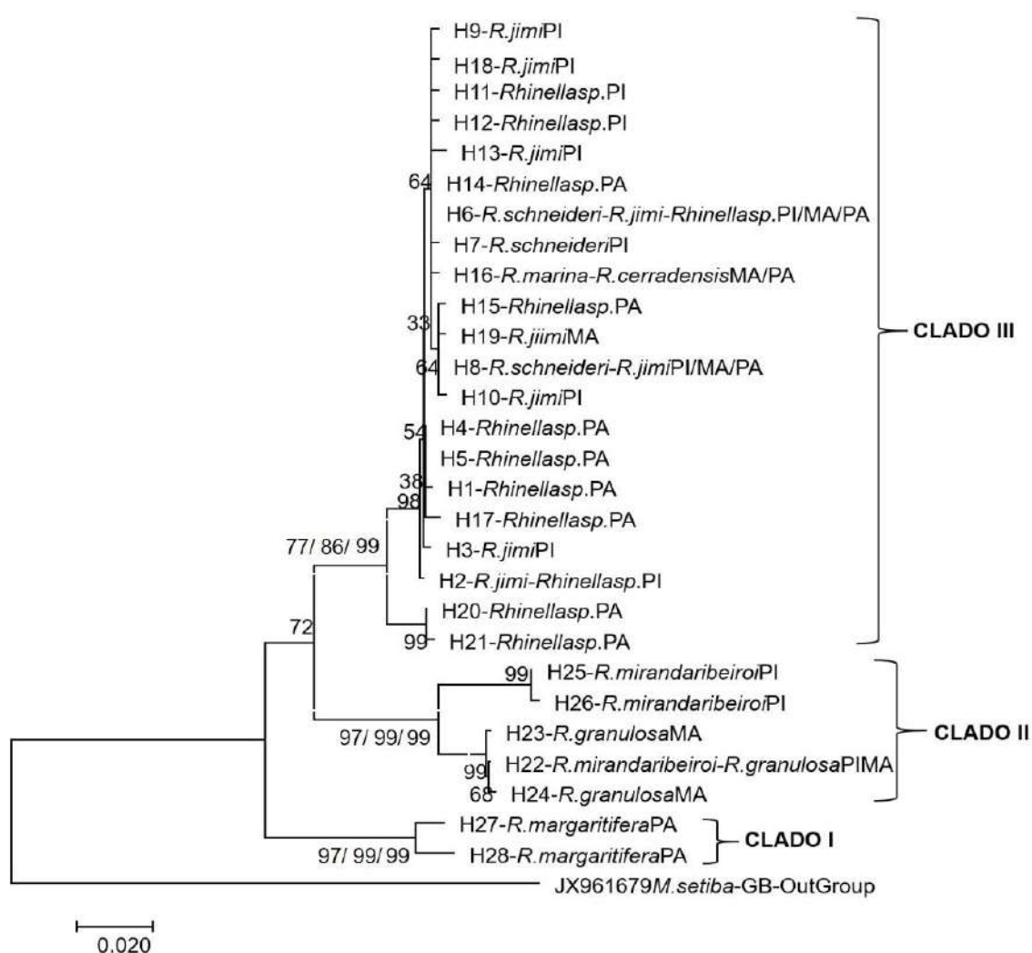
Figura 3. Árvore filogenética obtida através da abordagem de agrupamento de vizinhos (NJ) usando o algoritmo Tamura-3 Parâmetro para haplótipos do gênero Rhinella do meio norte do Brasil, com base no gene rRNA 16S. Os valores de bootstrap estão na seguinte ordem: Máxima Verossimilhança (ML), Máxima Parcimônia e Agrupamento de Vizinhos (NJ).
