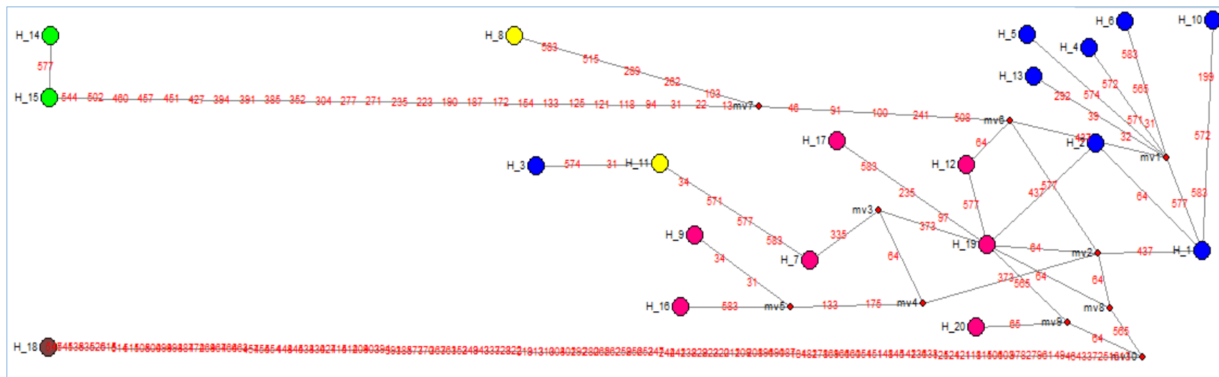
Figura 6. Rede de haplótipos gerada pelo programa network, mostrando as espécies identificadas pelo gene COI, na plataforma BLAST. As cores representam as espécies da seguinte forma: vinho= R. mirandaribeiroi ; Amarelo= R. schneideri ; Verde= R. marina . Azul = R. jimi ; róseo= R. ornata
