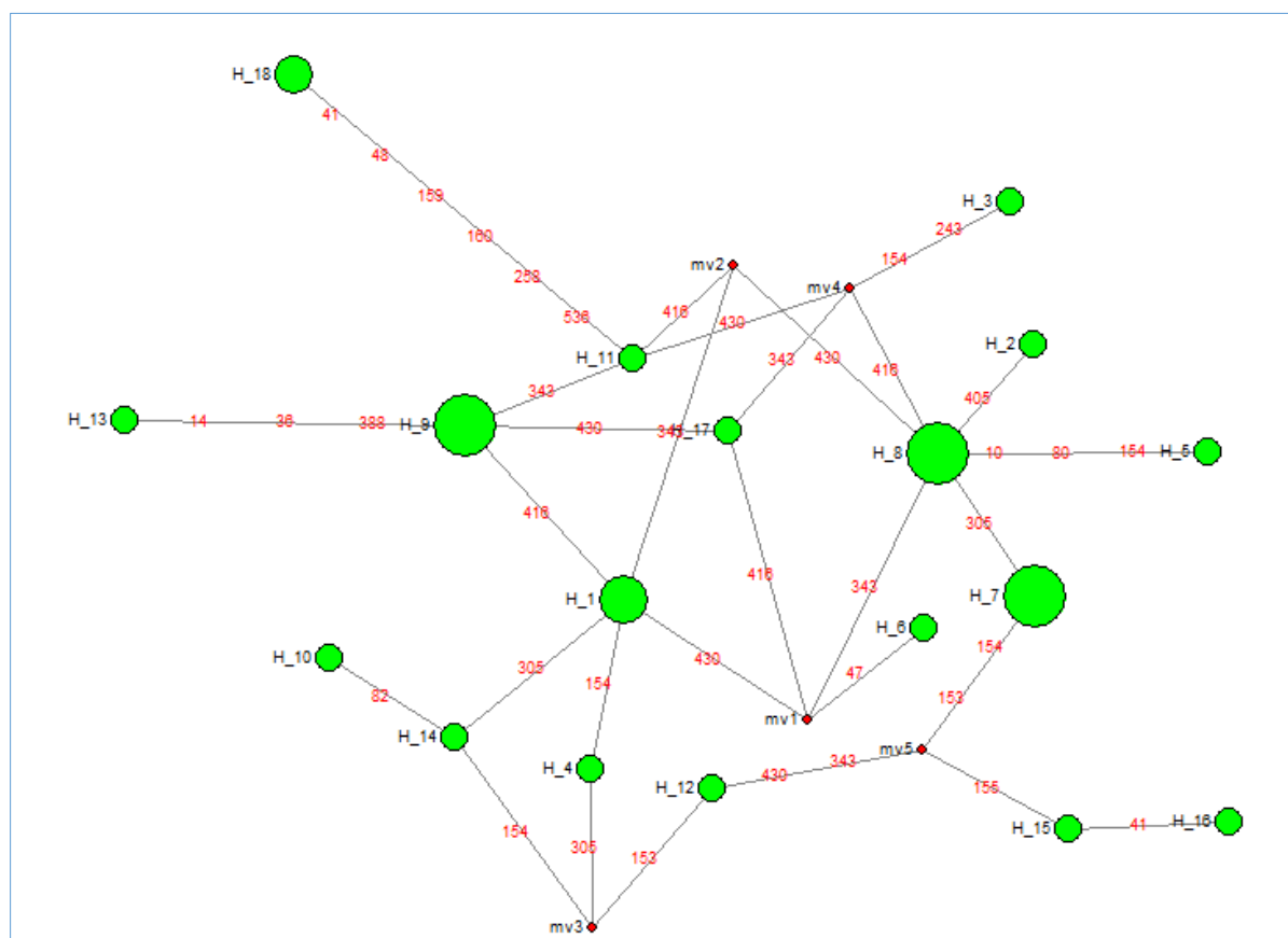
Figura 8. Rede de haplótipos gerada pelo programa network, mostrando a espécie identificadas pelo gene RPL35 na plataforma BLAST A cor representa a espécie R. marina .
